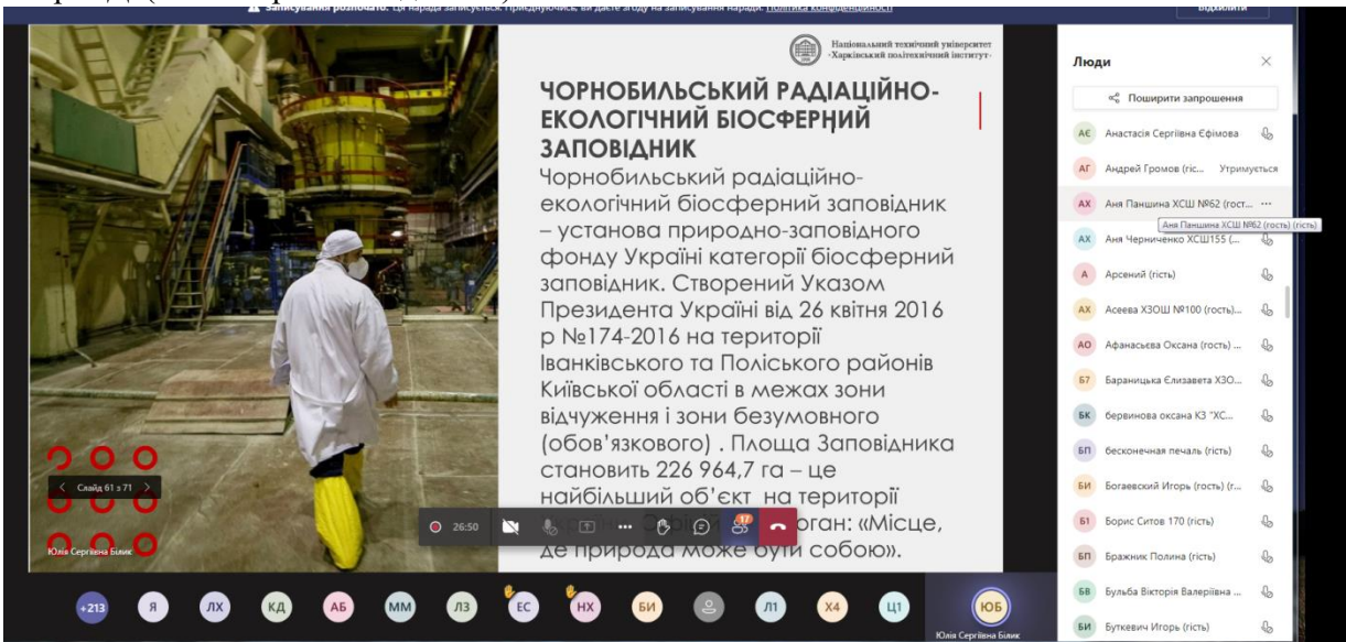
Паншина А.
