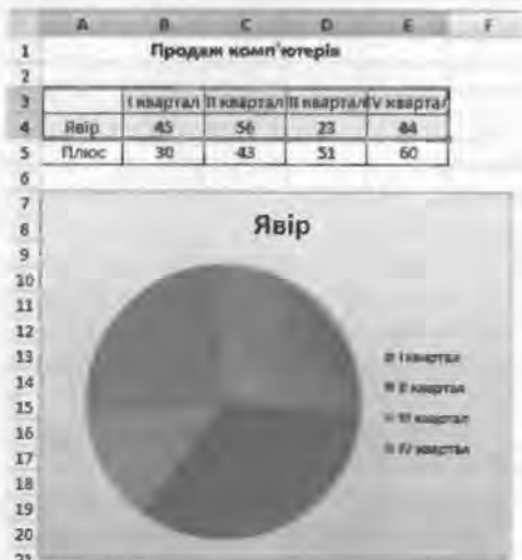
Рис. 2.66. Секторна діаграма
