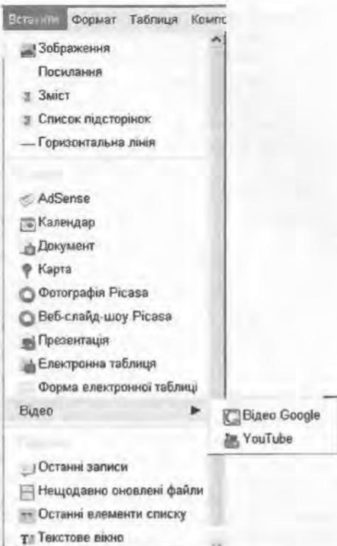
Рис. 4.36. Меню Вставити
