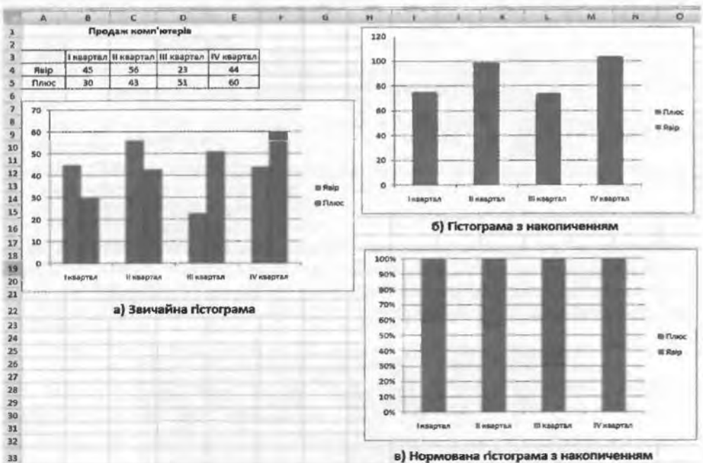
Рис. 2.64. Гістограми
